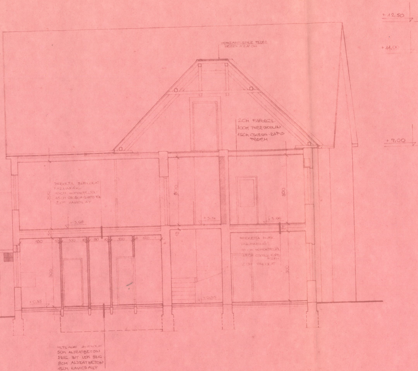
b-b metszet
